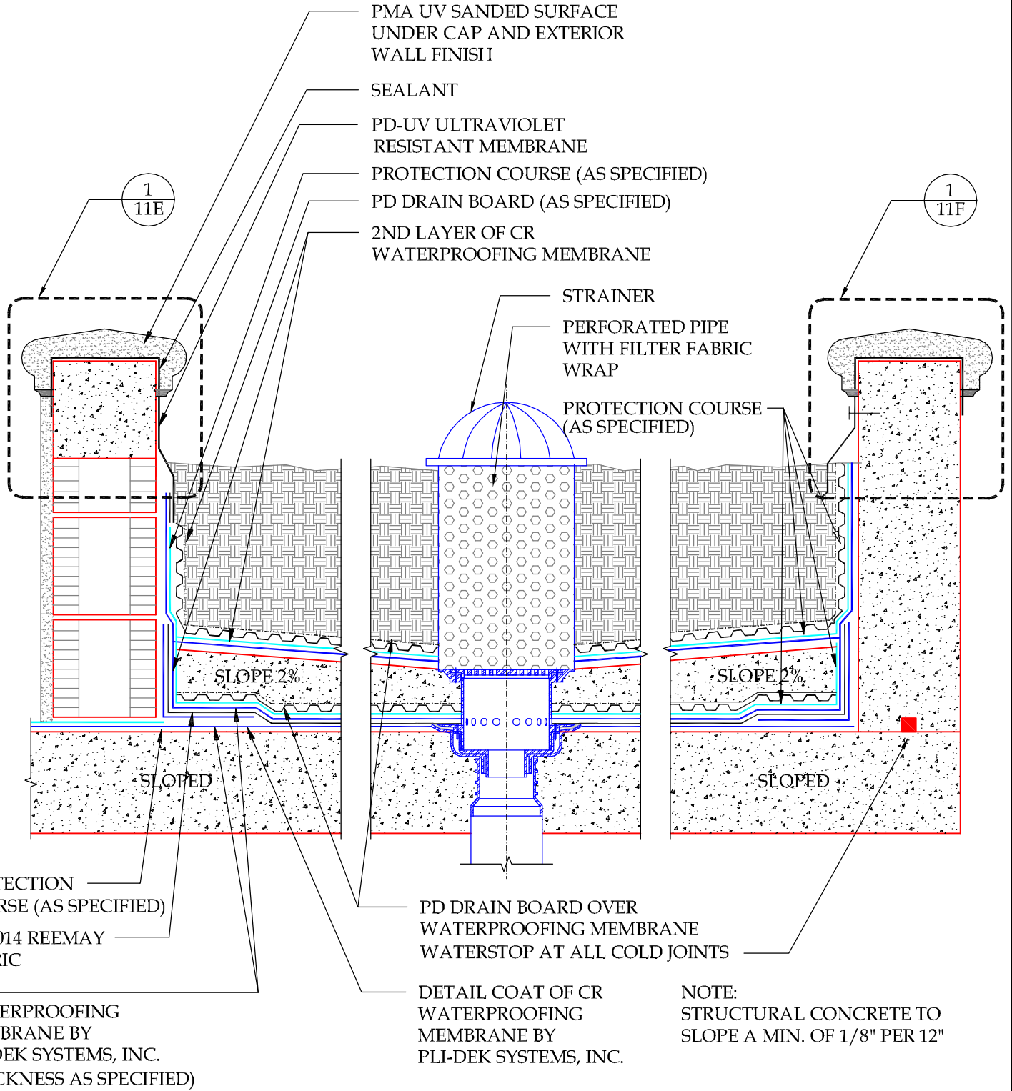
DETAIL-PLAZA DECK PLANTER SCALE: N.T.S.
