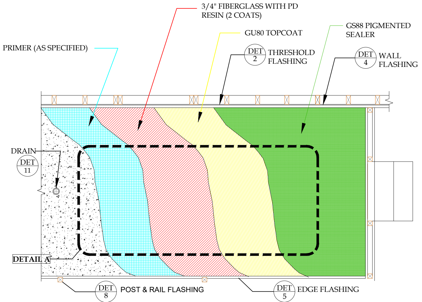
DETAIL-CON-DEK - DECK PLAN VIEW SCALE: N.T.S.
