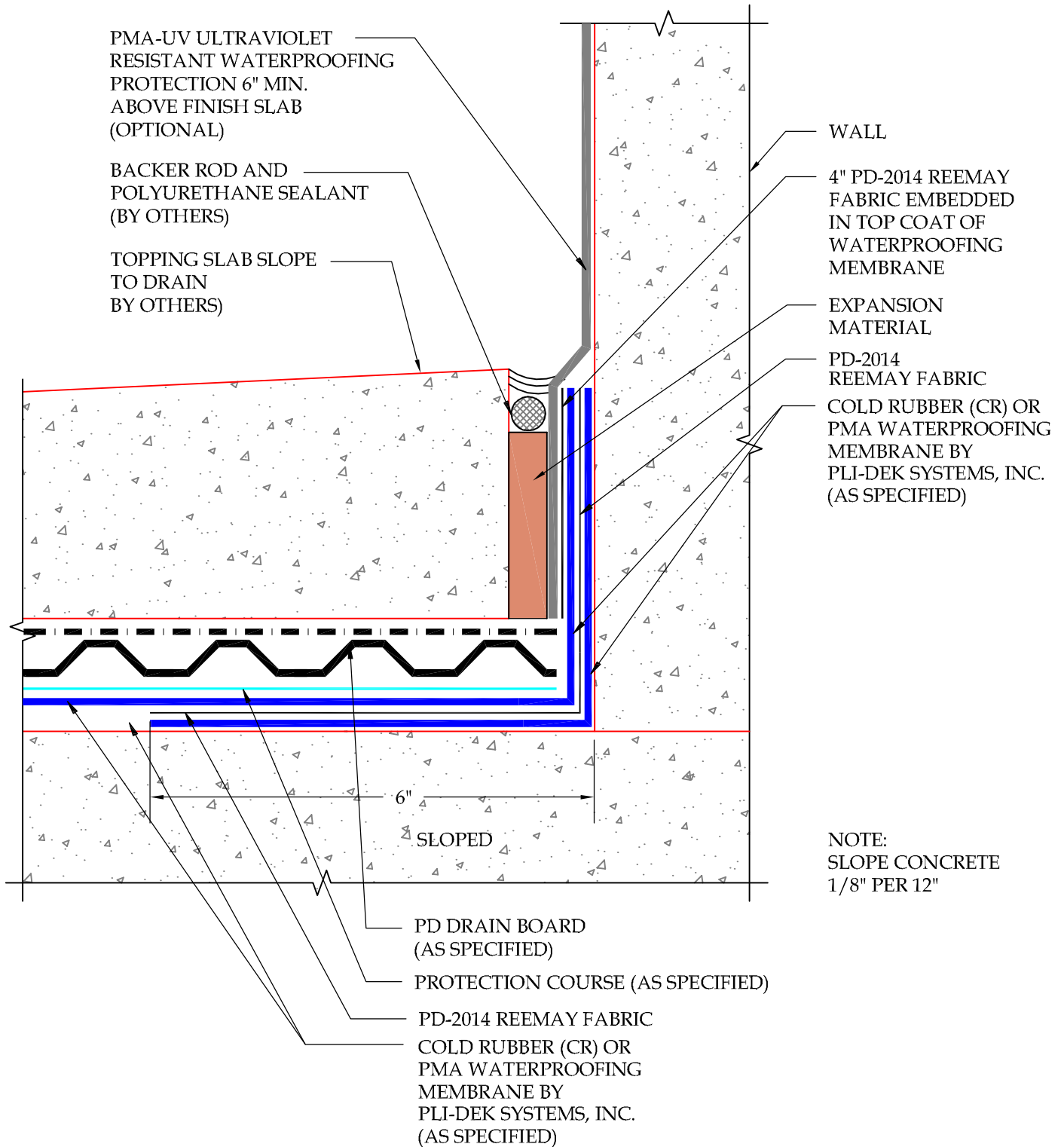
DETAIL-AT WALL JUNCTION SCALE: N.T.S.
